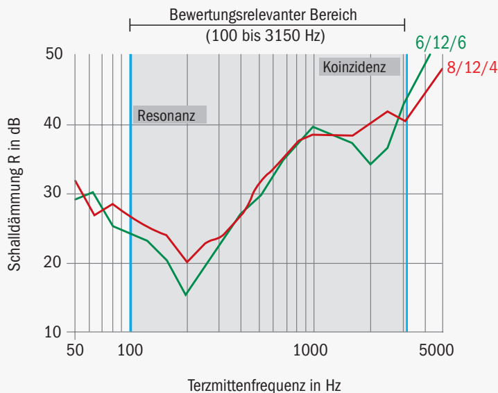
Abbildung 8: Oben: Schalldämmung in Abhängigkeit von der Frequenz Unten: Koinzidenz und Resonanz – Vergleich eines asymmetrischen und symmetrischen MIG-Aufbaus
