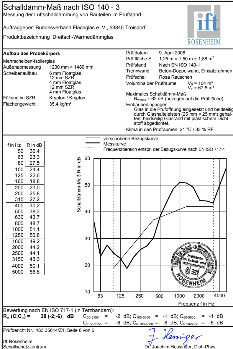
Abbildung 3: Musterprüfbericht für ein 3-fach Mehrscheiben-Isolierglas
