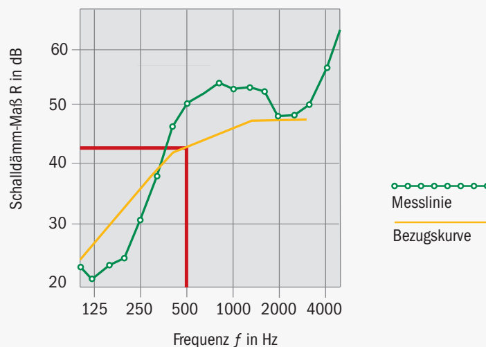
Abbildung 1: Ermittlung des bewerteten Schalldämm-Maßes nach DIN EN ISO 717-1
