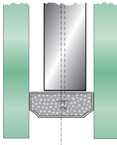
Abbildung 2: Sprossenlage
