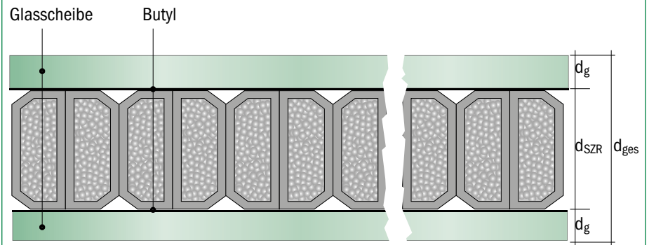
Abb. 6: Aufbau der Probekörper zur Messung der äquivalenten Wärmeleitfähigkeit eines Abstandhalters nach ift-Richtlinie WA 17/1 [5]
